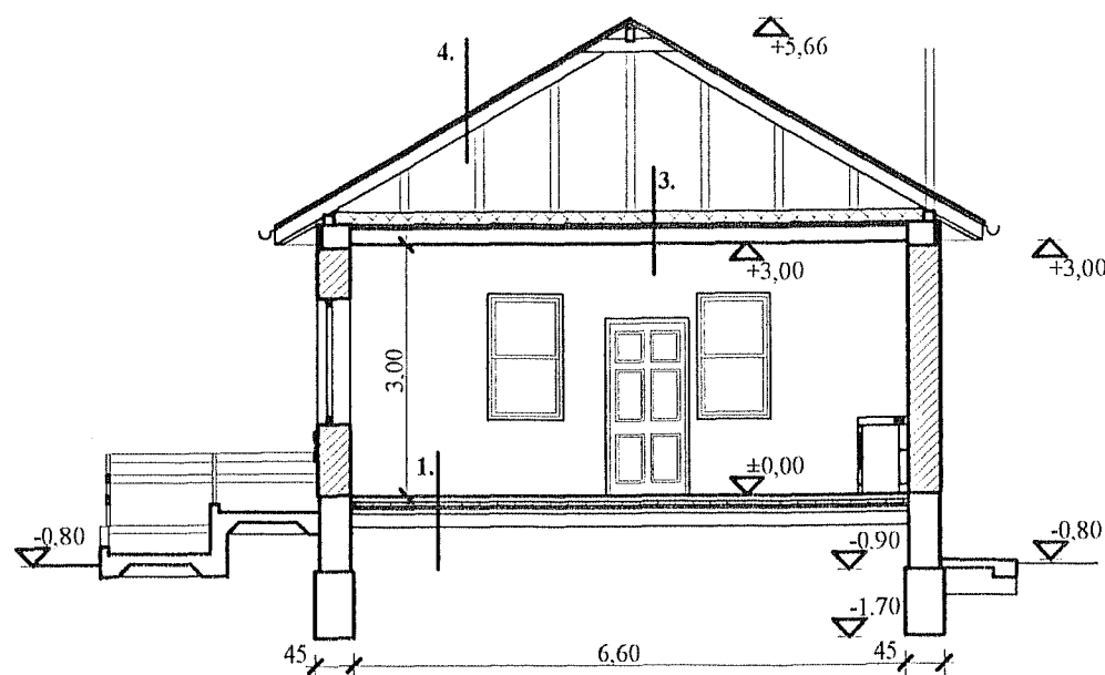
A - A METSZET M = 1 : 100
