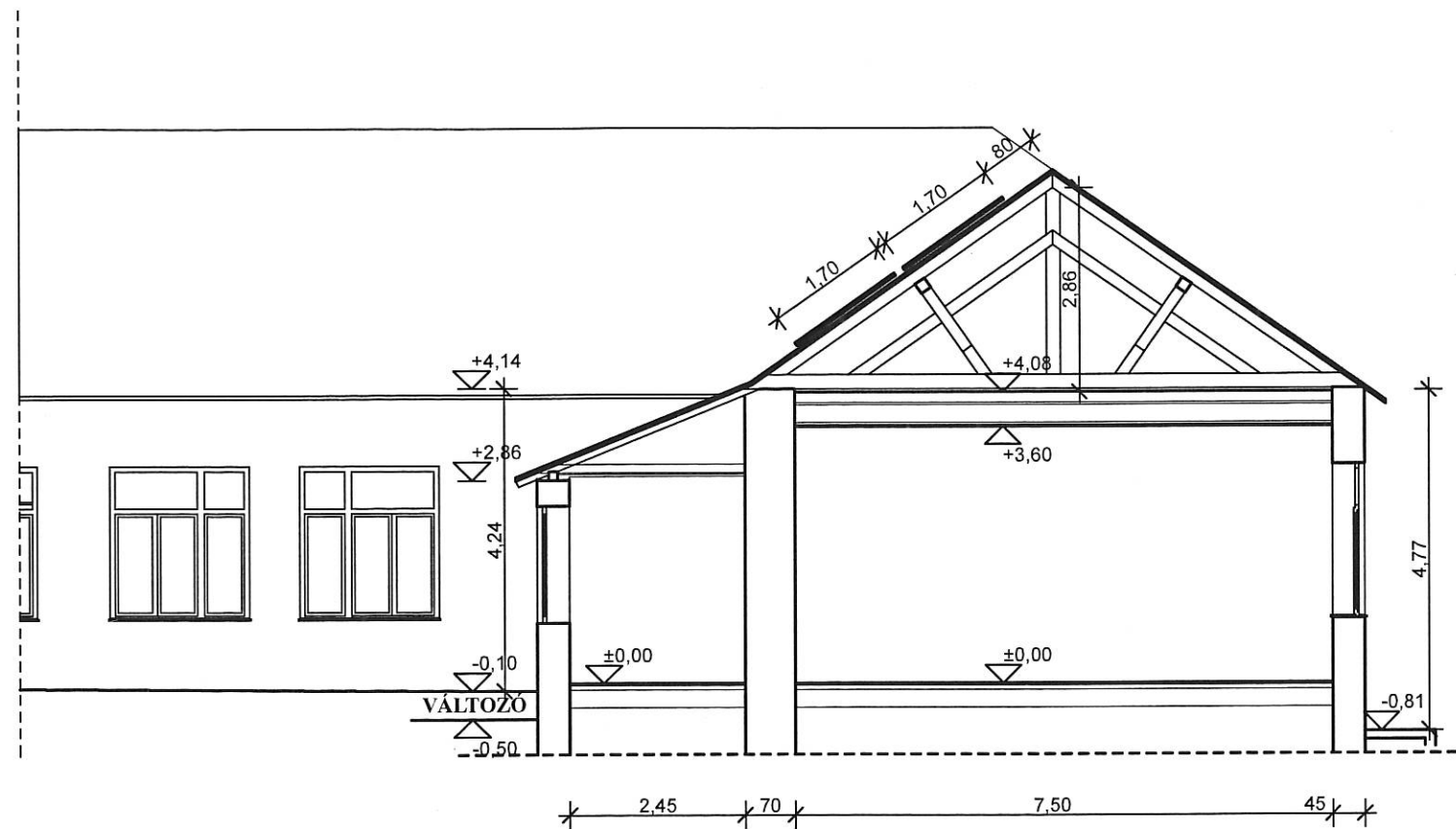
A - A METSZET M = 1 : 100
